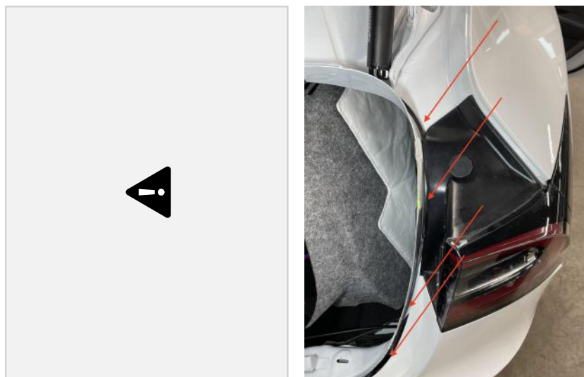
Abbildung 5: Hubarmkabel entlang der Kontur
