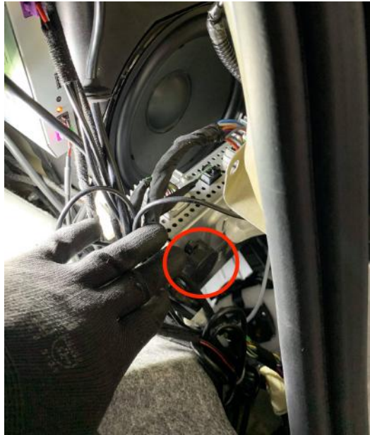
Abbildung 25: Anbringung des akustischen Signalgebers
