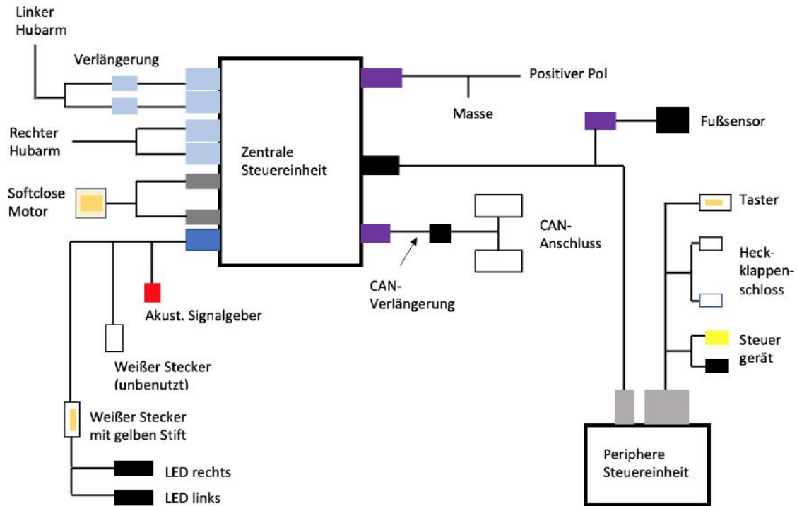
Abbildung 26: Systemaufbau
