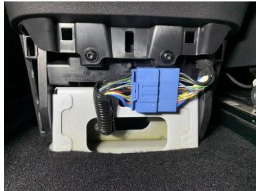
Abbildung 21: Abdeckung (links), CAN-Kabelbaum (rechts)
