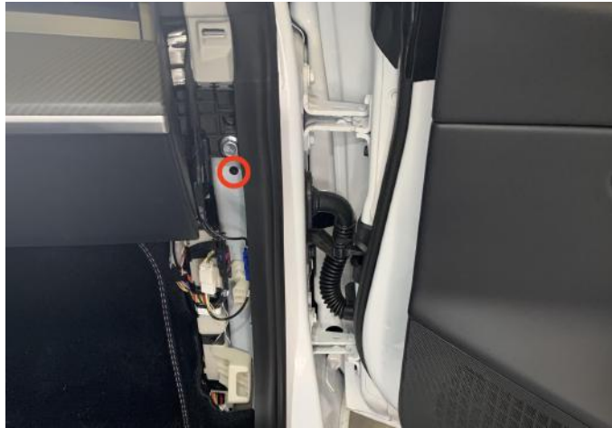
Abbildung 17: Befestigungsklemme seitlich des Armaturenbretts
