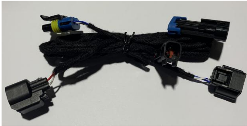
Abbildung 18: Kabelbaum Schließeinheit
