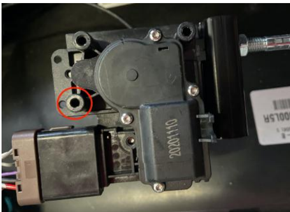
Abbildung 14: Öffnung für das Gewinde drehen (links) und Schraubbefestigung des Bowdenzugmotors (rechts)
